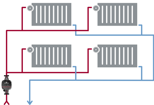
Двотрубна система опалення
