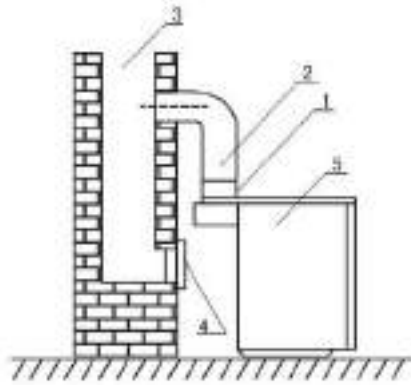
Малюнок 43. Орієнтовна схема підключення апарату до цегляної димоходу 1. димовідвідної патрубков апарату; 2. З'єднувальний патрубок; 3. Димохід; 4. Дверцята для чищення; 5. Апарат.
